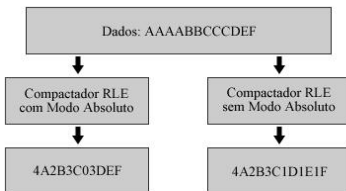
Figura 2.1 – Codificação de Run-Length Encoding Fonte: Friedrich, 2004.
