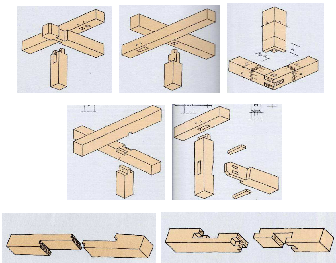
Figura 51 – Outros encaixes utilizados na marcenaria.
