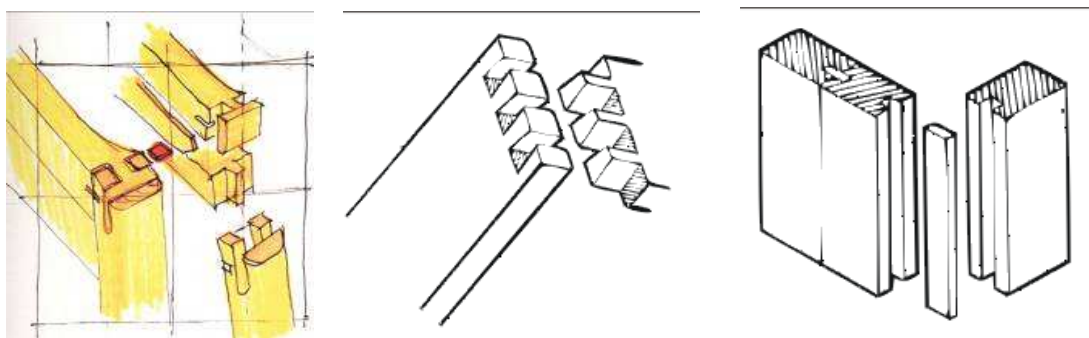
Figura 52 – Encaixes utilizados por Maurício Azeredo.
