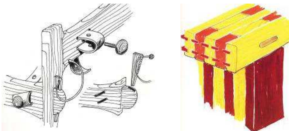
Figura 46 – Sistemas de Encaixes utilizados pelos autores.
