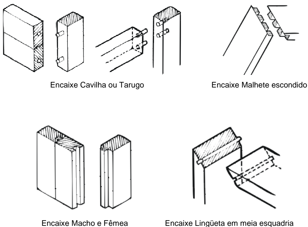
Figura 50 – Encaixes mais utilizados na marcenaria
