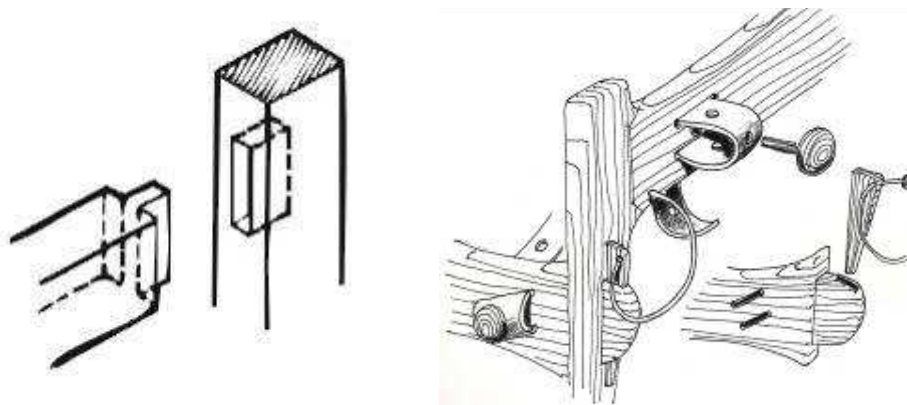
Figura 53 – Encaixes utilizados por Sérgio Rodrigues.
