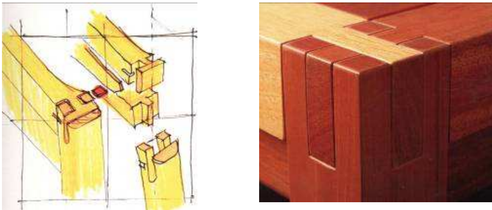
Figura 37 - Junta Tridimensional.
