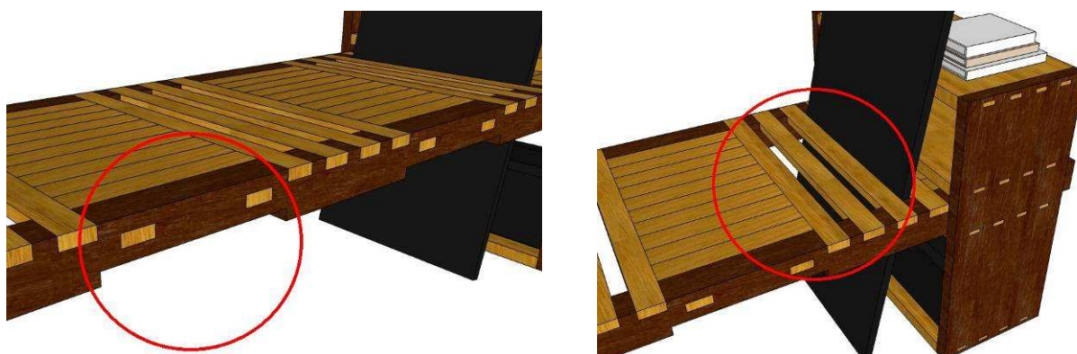
Figura 60: Encaixe para nichos e prancha vertical.
