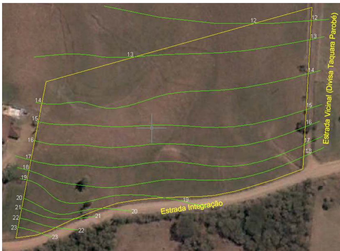
Imagem 9 – Levantamento Topográfico do terreno
