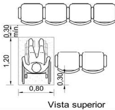
Imagem 10 — Espaçamento para P.C.R. na última fileira (Fonte: NBR9050, 2004)
