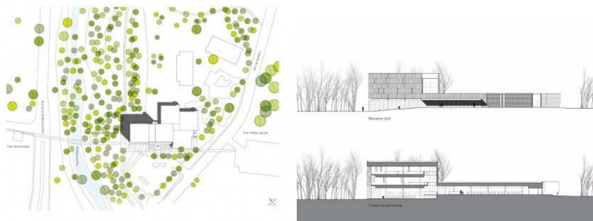
Figura 8 – Implantação da Biblioteca Montarville e Figura 9 – Corte da Biblioteca Montarville Fonte: CONCURSODEPROJETO, 2010.
